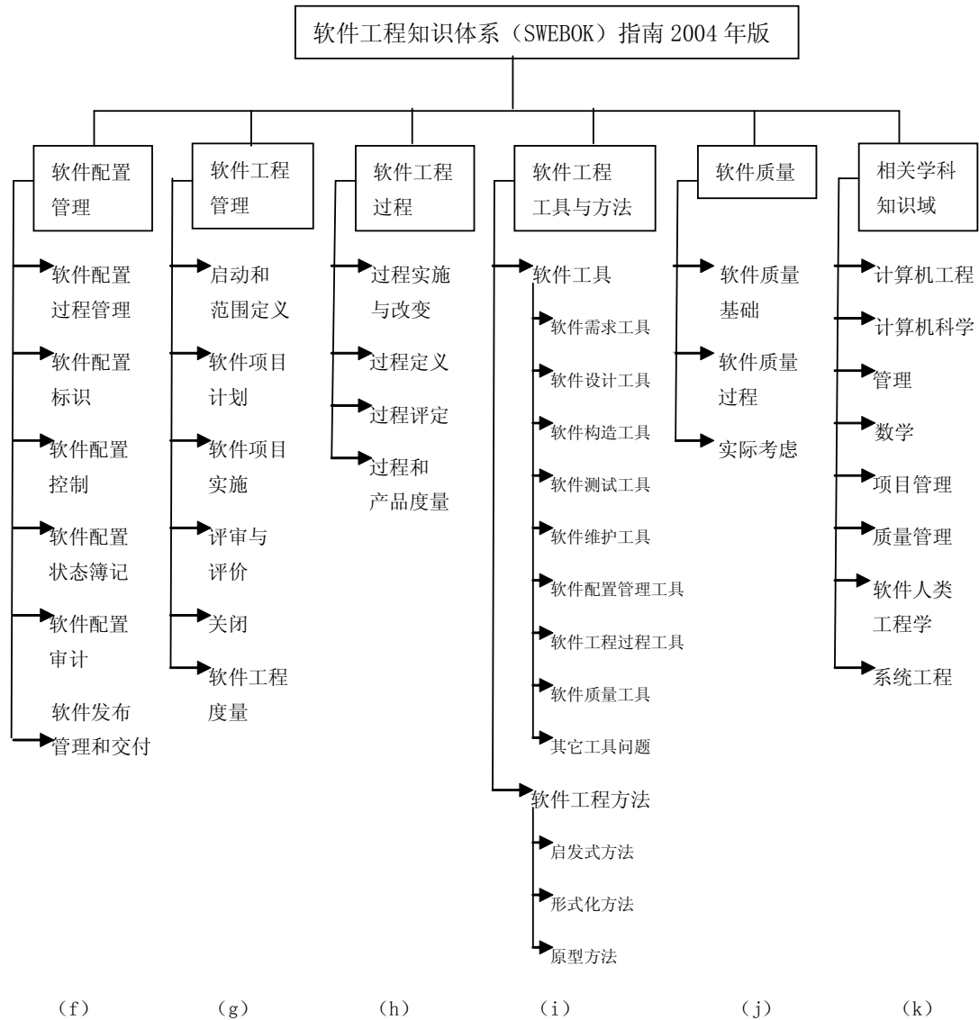
图3 后6个知识域
