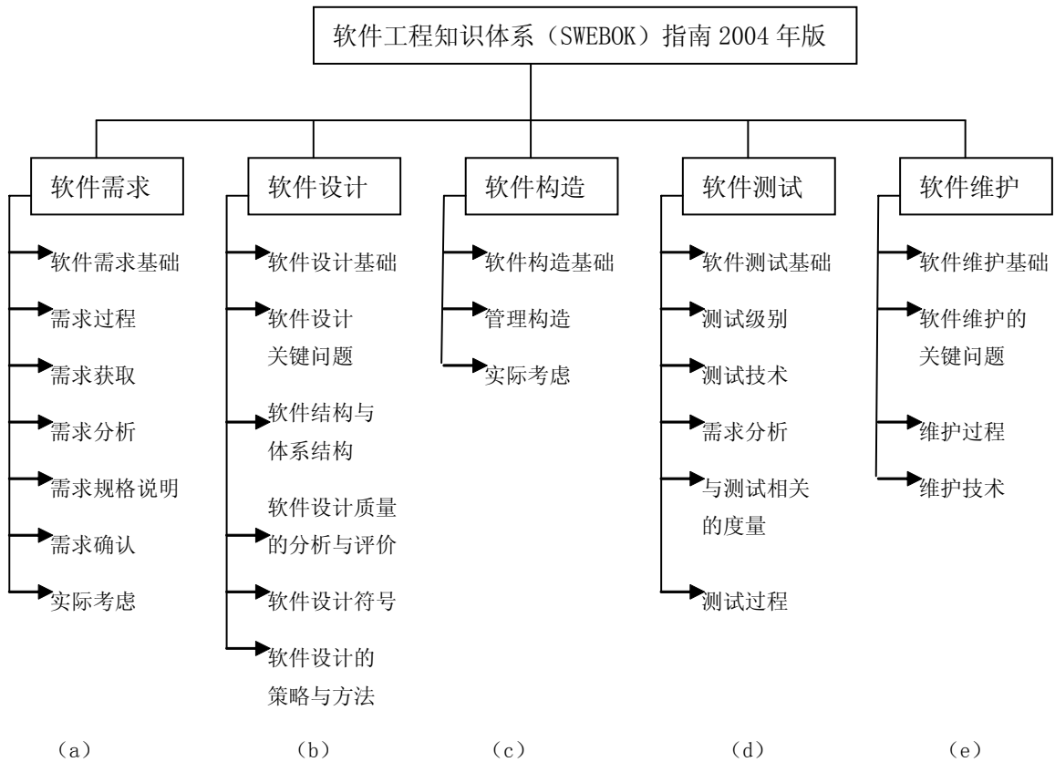
图2 前5个知识域
